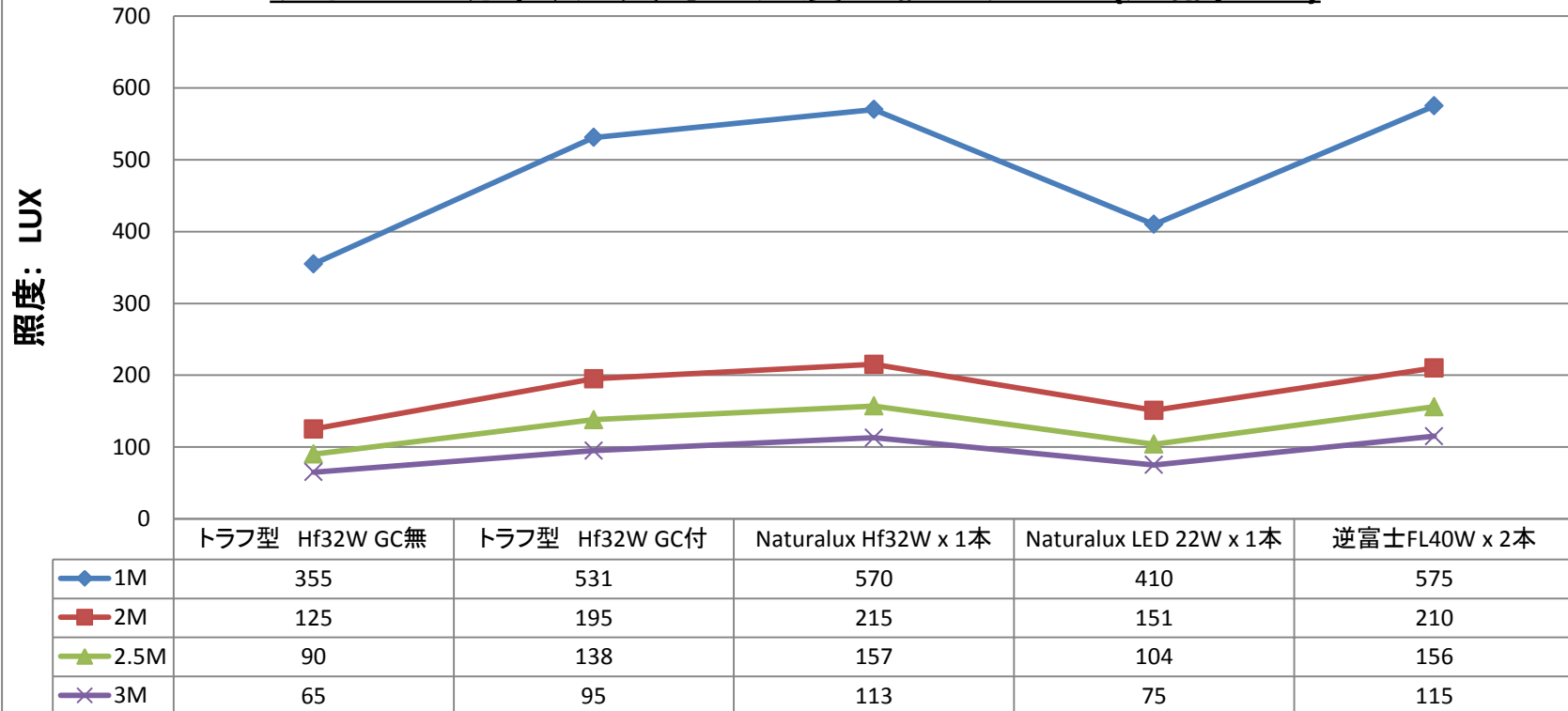
反射笠の効果、灯具毎の照度比較グラフ (距離/LUX)
